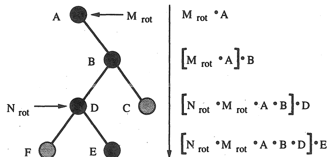
Figura 4: Expansão da composição de transformações em uma estrutura articulada hierárquica.
